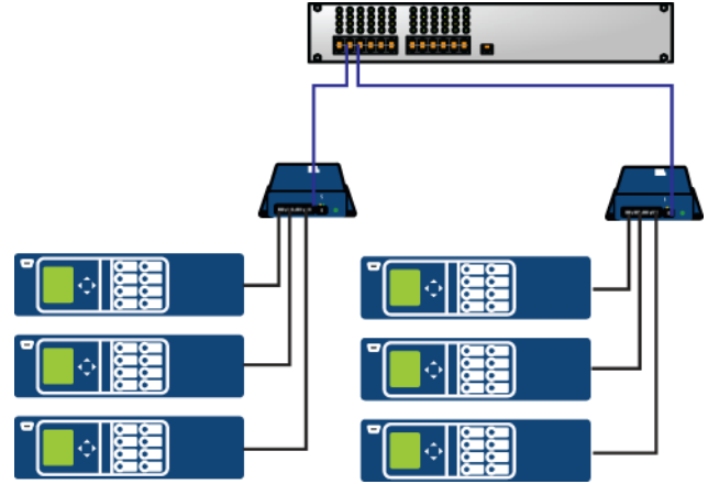
Fig. 12. Substation LAN
